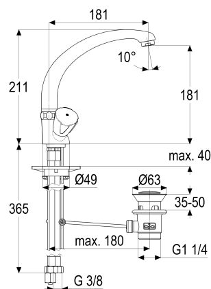
Maßzeichnung
