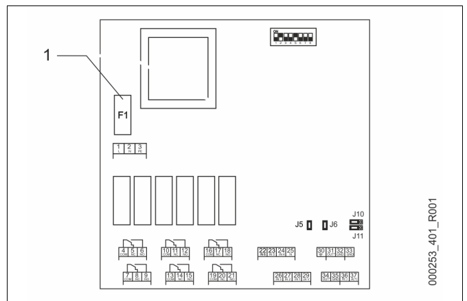
1 Feinsicherung F1 (250 V, 0, 16 A träge)
