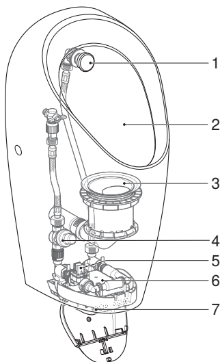
Зображення 1: Пісуари Geberit Selva, Preda й Tamina з інтегрованою системою керування та роботою від мережі
