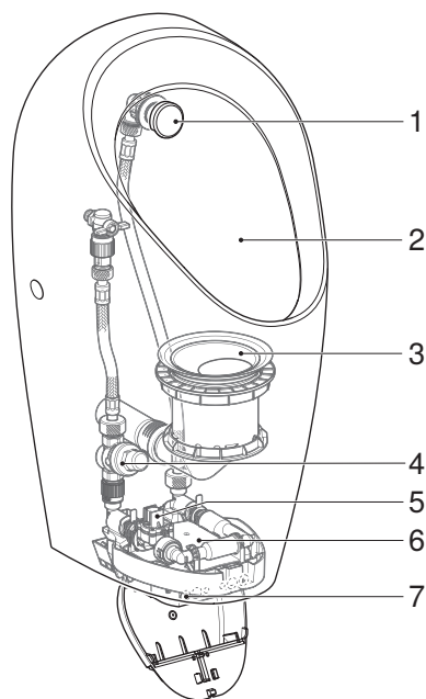
Ilustrimi 1: Pisuaret Geberit Selva, Preda dhe Tamina me njësi komandimi të integruar, funksionim elektrik
