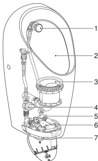
Илустрација 1: Geberit писоари Selva, Preda и Tamina со вграден контролер, мрежна работа
