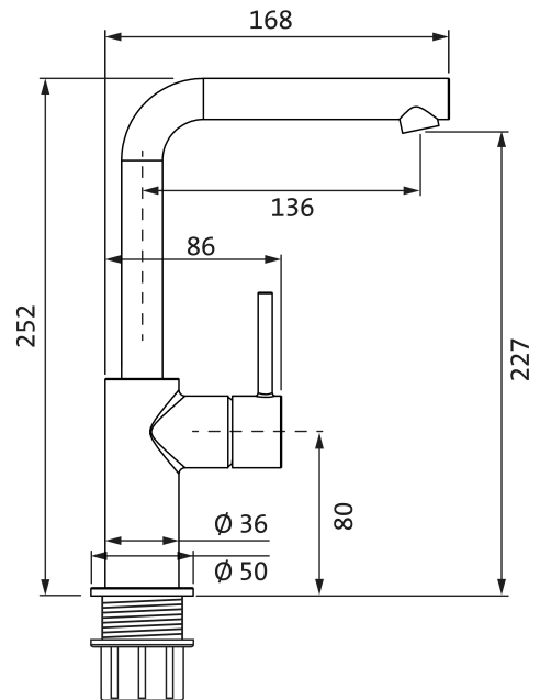
Lochbohrung Ø 35 mm hole diameter
