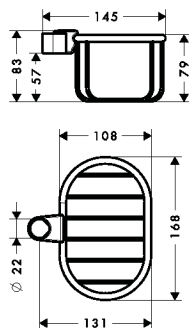
AXOR Montreux 42066XXX
