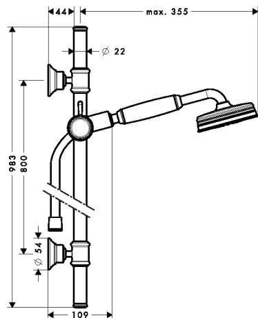
AXOR Montreux 27982XXX
