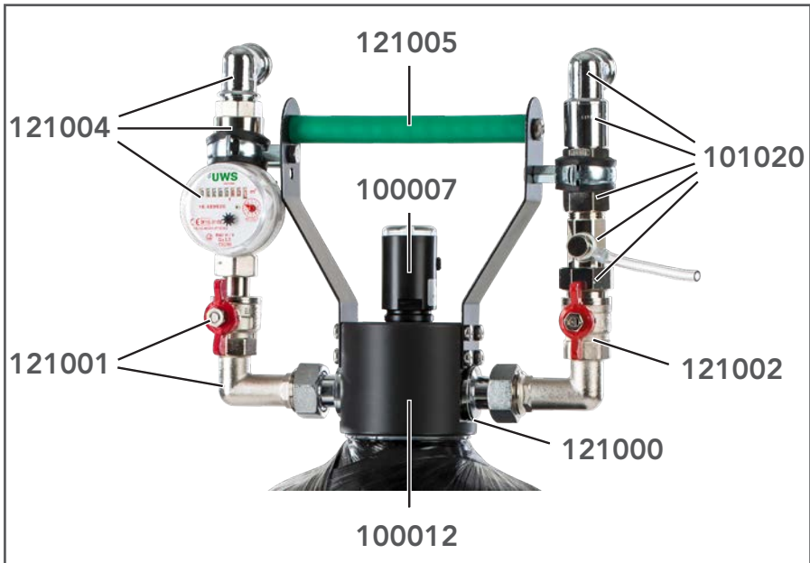
Bild 6-8: Ersatzteile Heaty Small 100 HW
