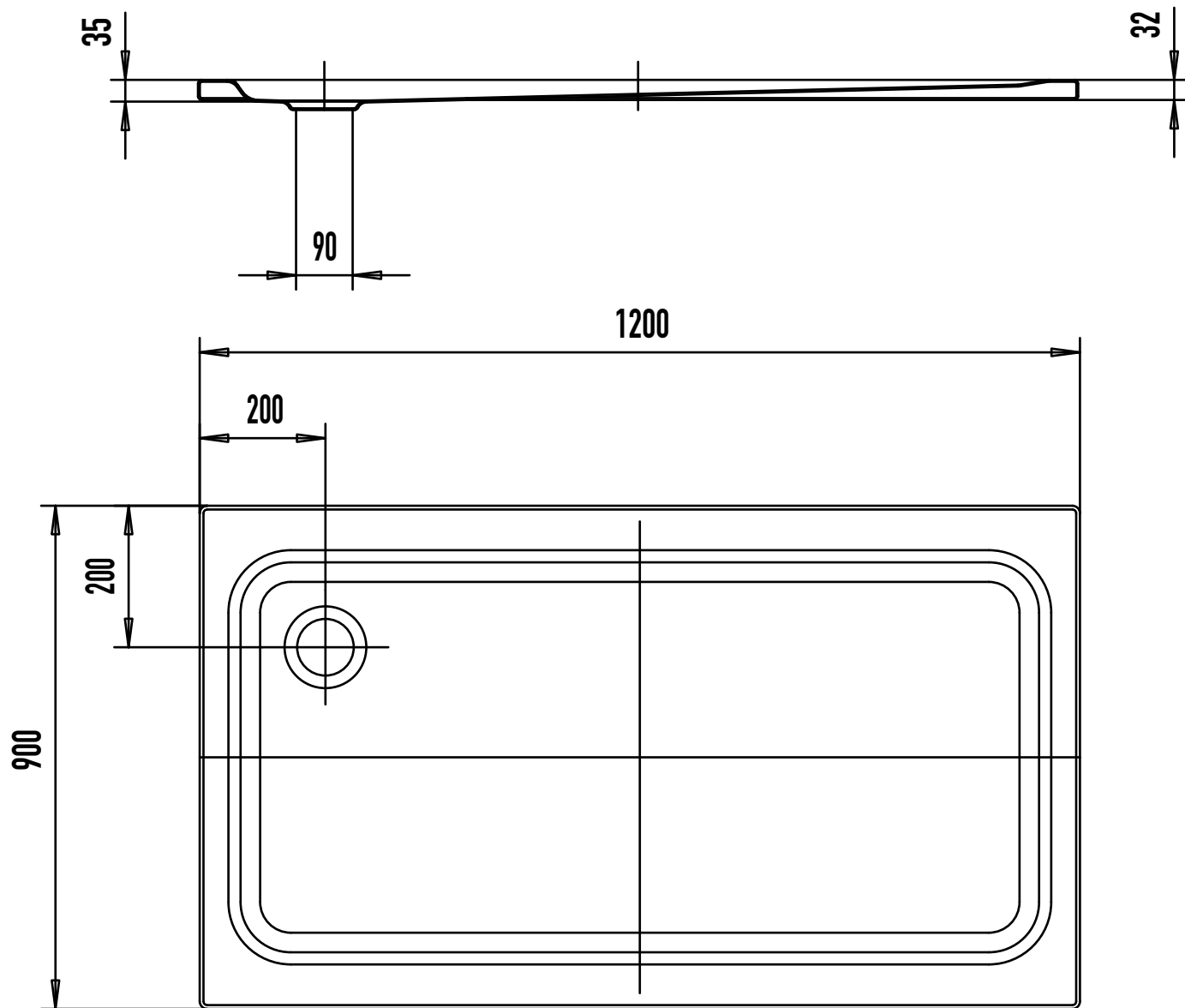
Duschwanne 1200 x 900 x 32 mm
