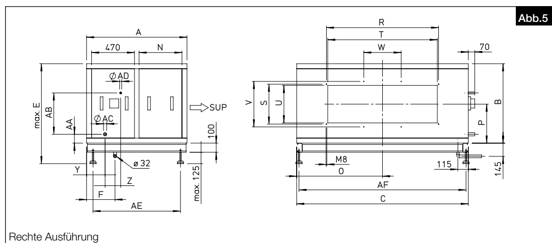
Abmessungen Change-Over-Register DX XH 1000-8500
