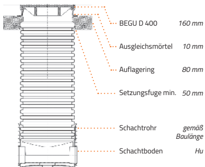
Betonaufagerung mit handelsüblicher Gussabdeckung
