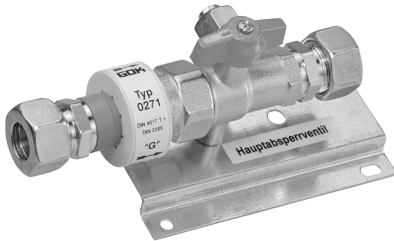
Type 0271 avant l'introduction dans l'habitation
