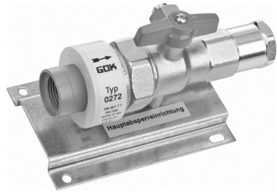
Type 0272 après l'introduction dans l'habitation
