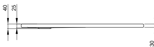
Duschwanne mit Schenkel ≤ 1000 mm
