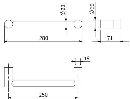
Maßzeichnung/ Dimensional drawing
