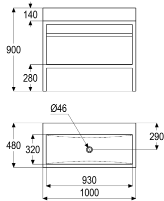
Maßzeichnung
