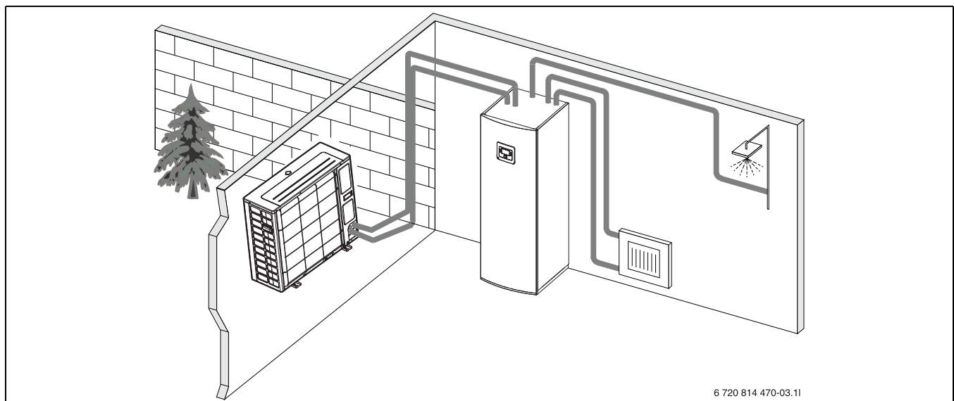
Bild 2 Wärmepumpe Außeneinheit, Inneneinheit ASM/ASMS mit integriertem Warmwasserspeicher und elektrischem Zuheizung
