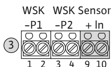
Fig. 12: Klemmleiste Sensorik: Anschluss Ni- veaufassung
