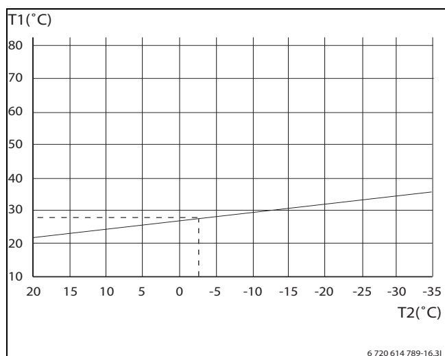
Bild 52 Fußbodenheizung
