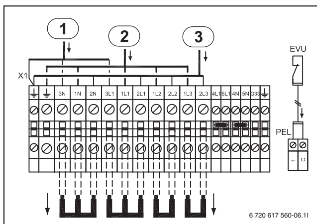
Bild 38 Alternative B, STE 60-1 - 100-1 und STM 60-1 - 100-1
