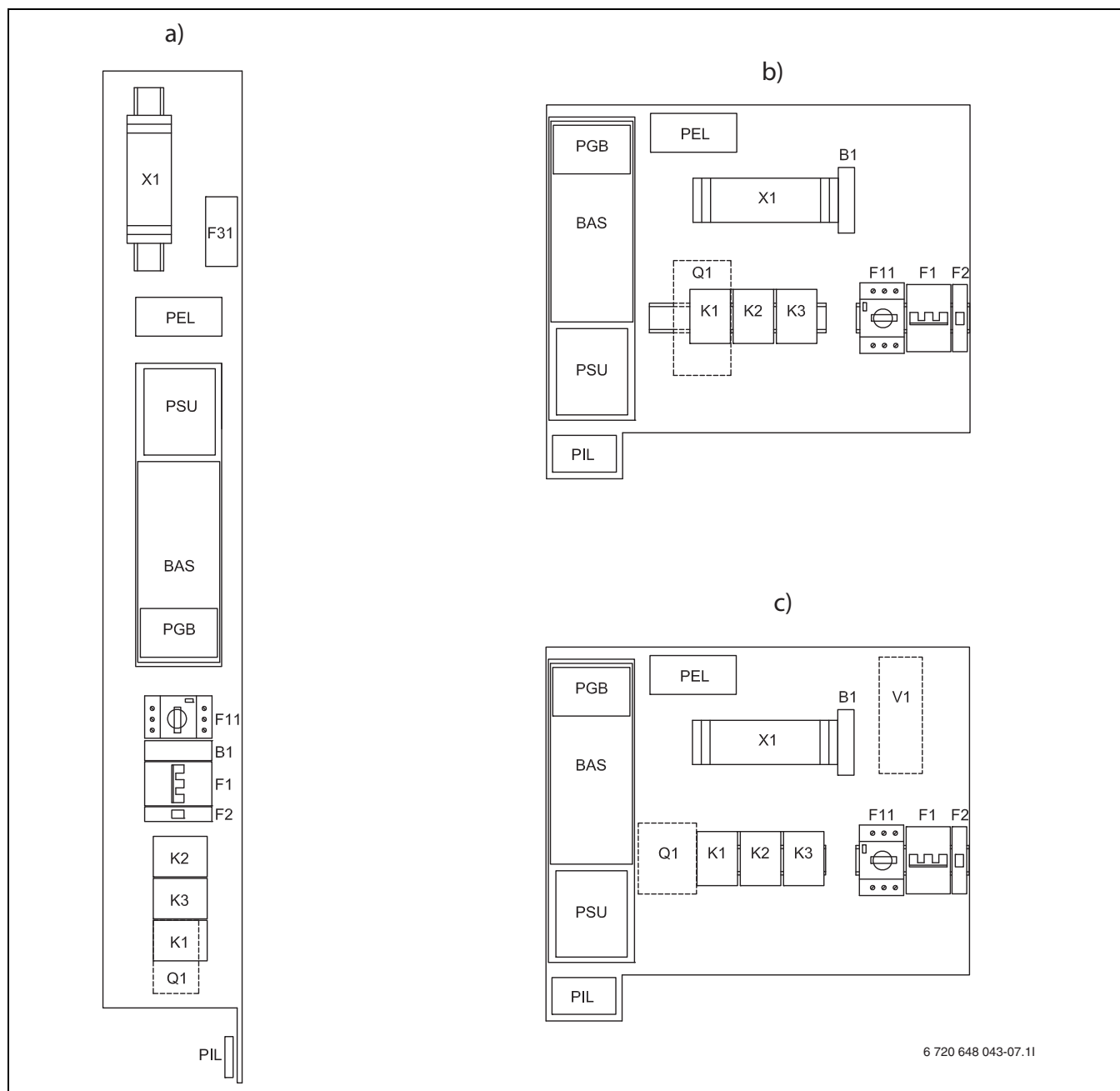
Bild 31 Übersicht Leiterplatte
