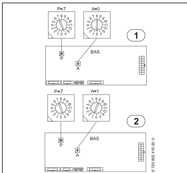
Bild 66 Adressierung von Wärmepumpe 1 und 2 bei Kaskadenschaltung.
