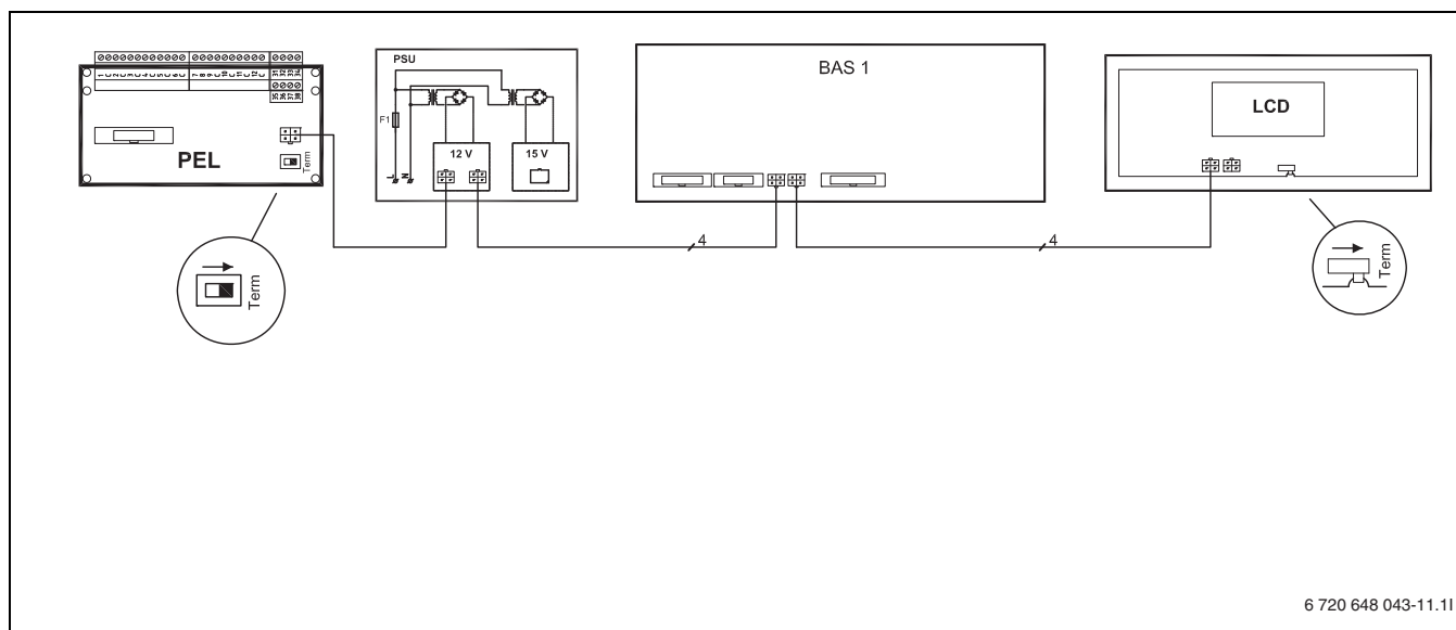
Bild 32 CAN-BUS-Übersicht
