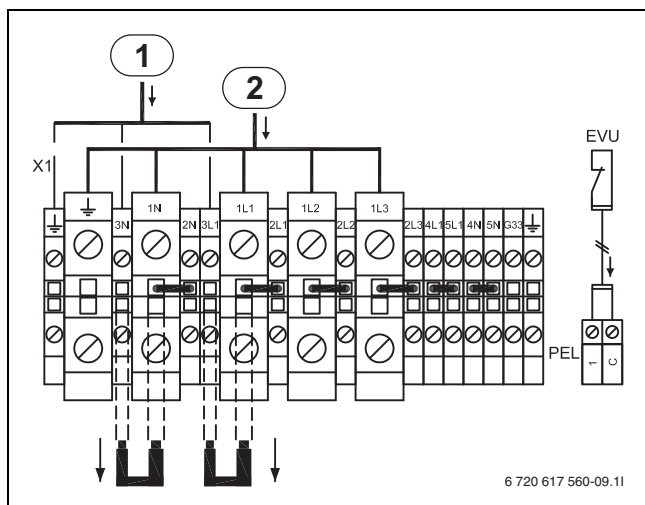
Bild 41 Alternative A, STE 130-1 - 170-1
