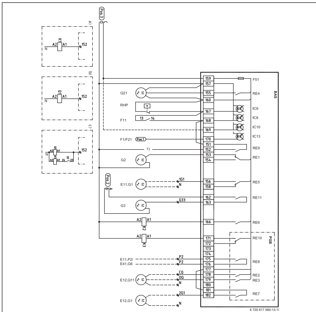
Bild 47 Kompletter Anschlussschaltplan (230 V)
