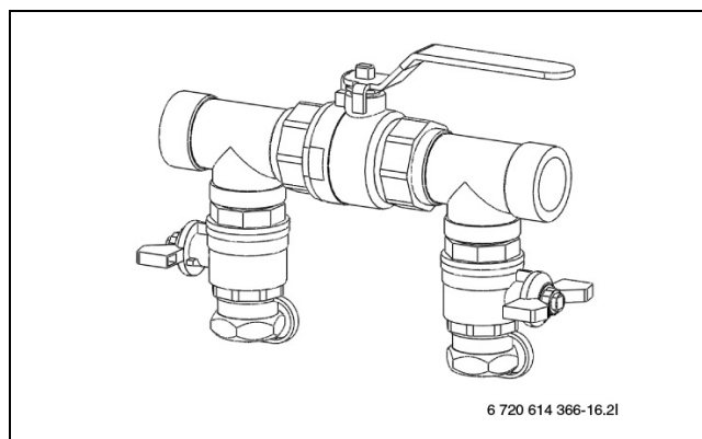
Bild 23 Befüllvorrichtung STE 130-1 - 170-1
