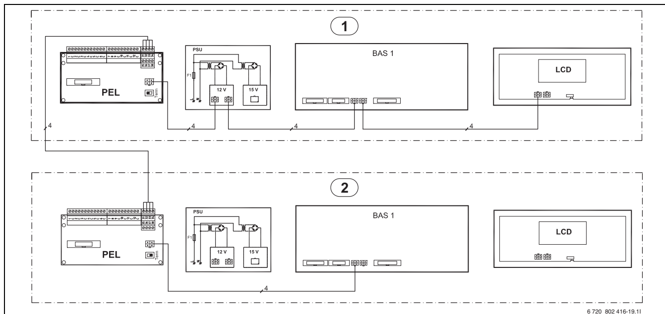
Bild 65 CAN-BUS-Übersicht mit zwei Wärmepumpen (6–17 kW)
