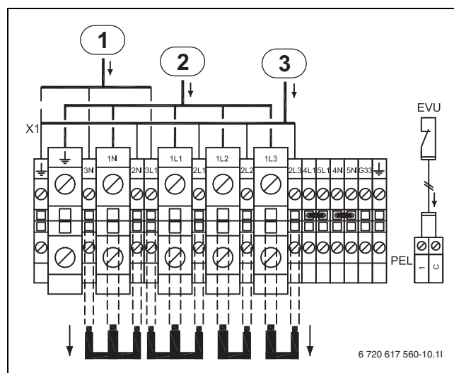
Bild 42 Alternative B, STE 130-1 - 170-1
