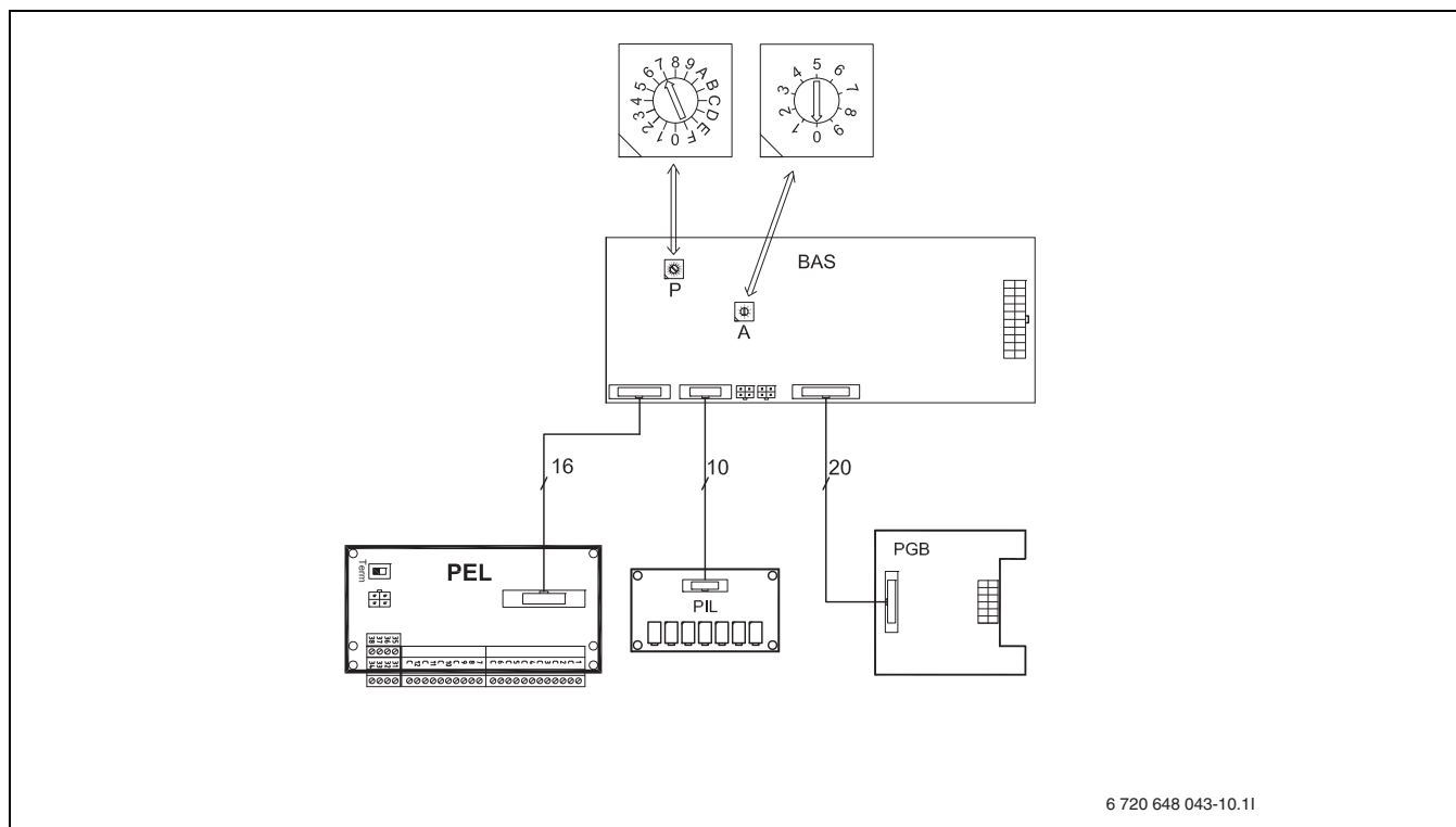
Bild 33 Leiterplattenverbindungen
