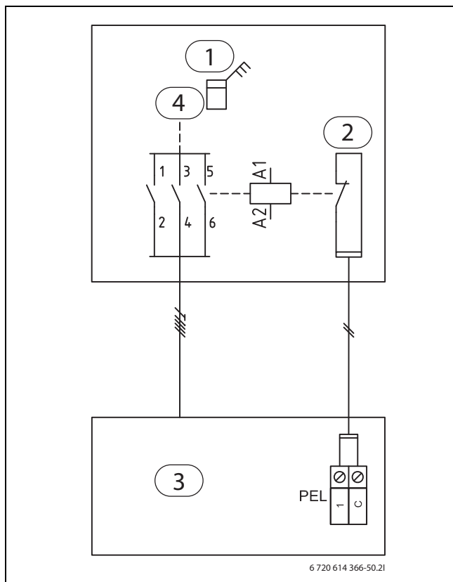
Bild 34 Sperrzeit aktiv
