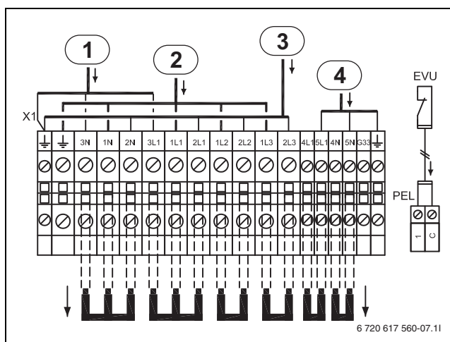
Bild 39 Alternative C, STE 60-1 - 100-1 und STM 60-1 - 100-1
