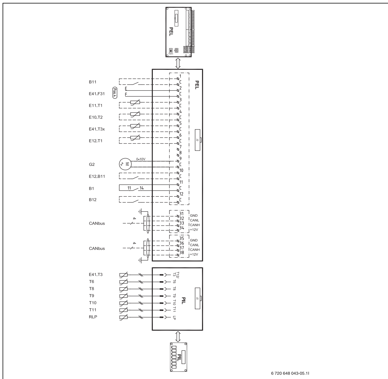
Bild 48 Kompletter Anschlussschaltplan (Niederspannung)
