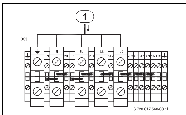
Bild 40 Standardausführung, STE 130-1 - 170-1
