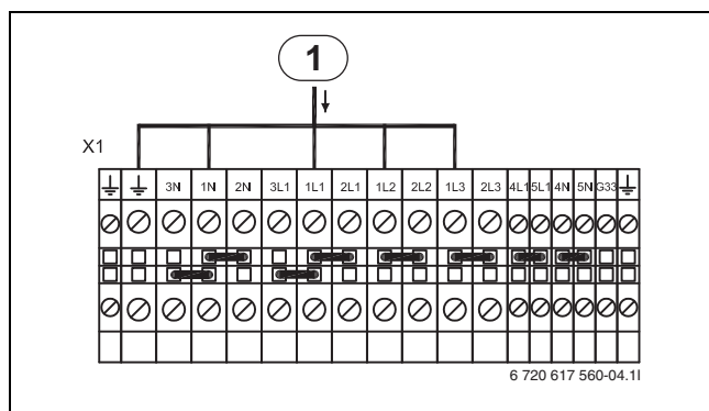
Bild 36 Standardausführung, STE 60-1 - 100-1 und STM 60-1 - 100-1
