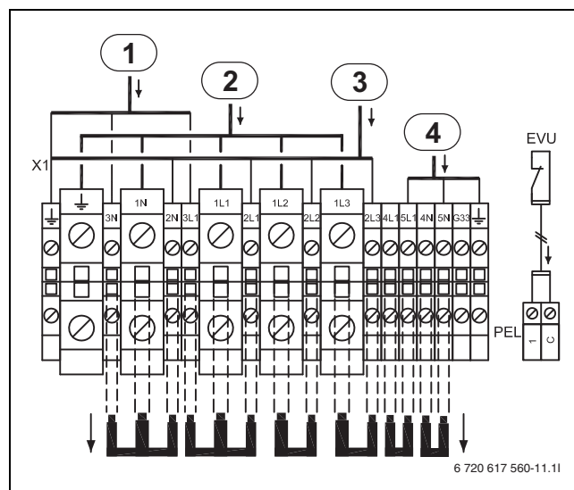
Bild 43 Alternative C, STE 130-1 - 170-1
