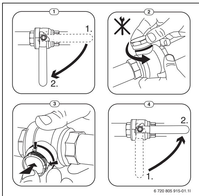
Bild 63 Filtervariante ohne Sicherungsring
