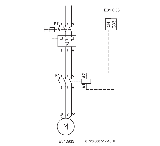
Bild 45 Anschluss Grundwasserpumpe
