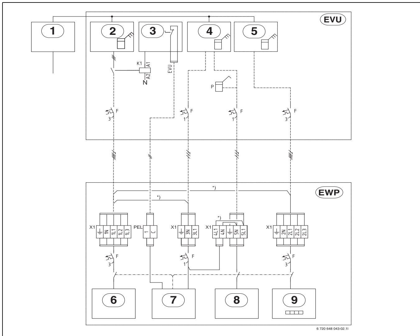
Bild 30 Anschlussübersicht Elektroschaltschrank - Wärmepumpe
