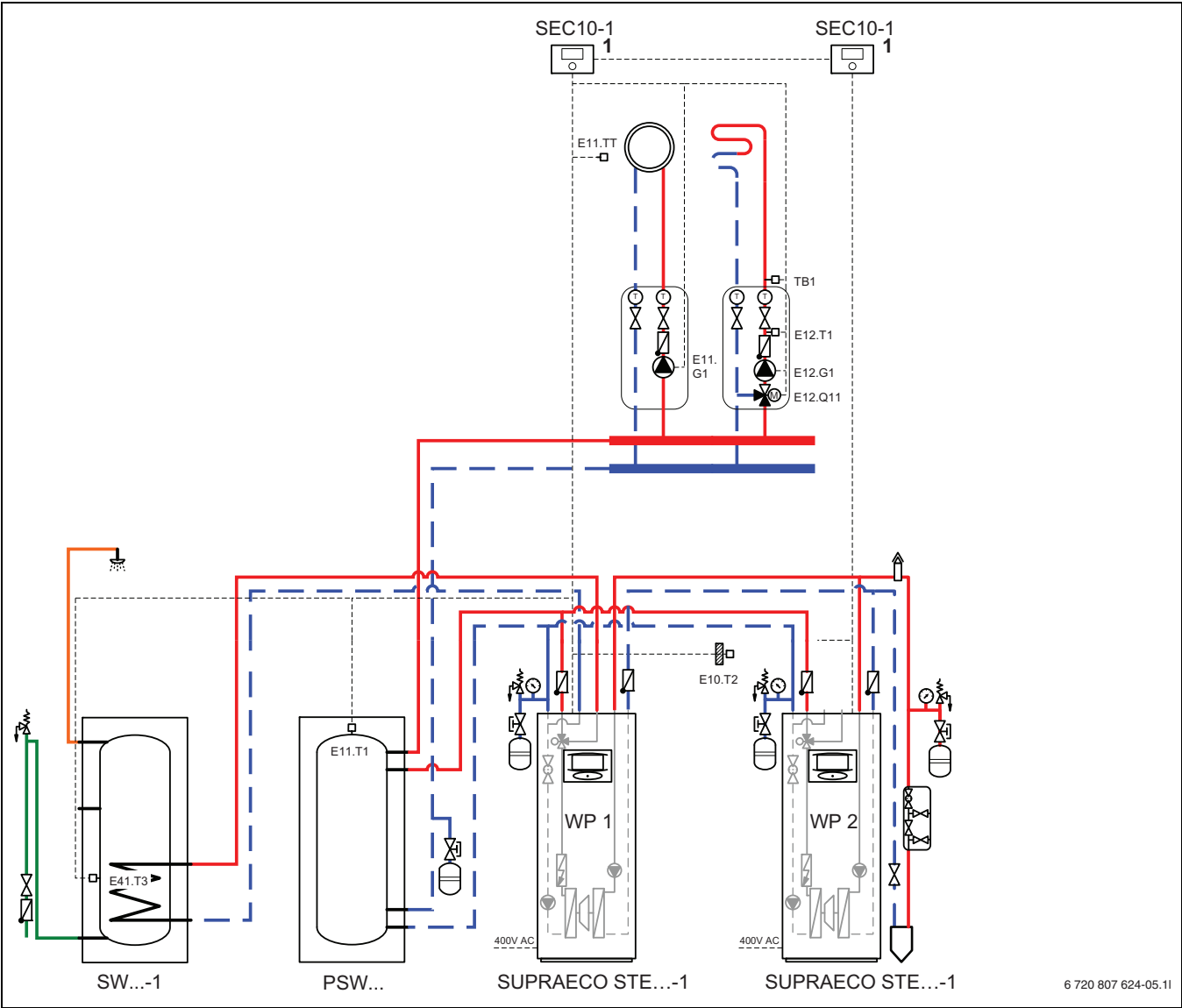
Bild 64 Zwei Wärmepumpen (Kaskadenschaltung) mit gemischtem und ungemischtem Heizkreis, Pufferspeicher und externem Warmwasserspeicher.
