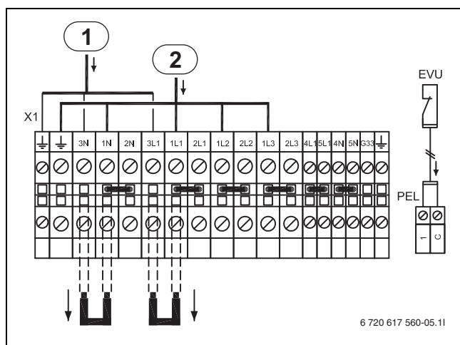
Bild 37 Alternative A, STE 60-1 - 100-1 und STM 60-1 - 100-1
