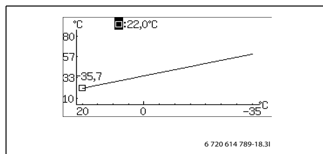
Bild 53 Einstellungsanzeige Heizkurve (Heizung)
