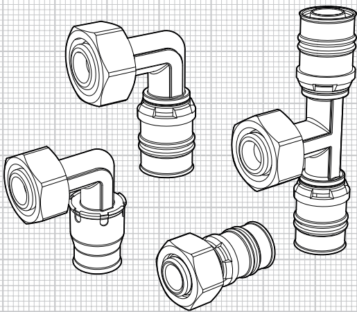
Messingverbinder Fix Anschluss Uni Brass adapter fix connector uni
