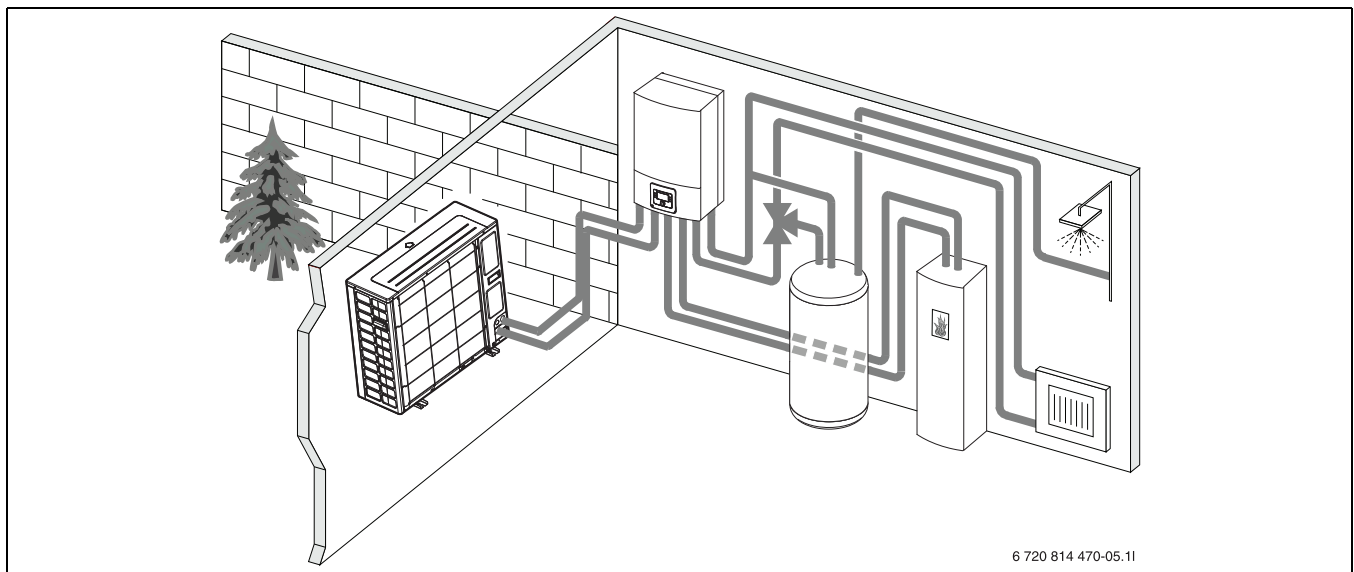
Bild 2 Wärmepumpe Außeneinheit, Inneneinheit ASB ohne elektrischen Zuheizler, externer Warmwasserspeicher und externer Zuheizler
