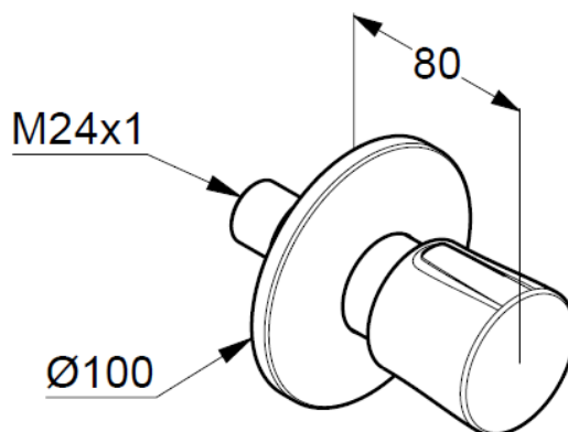
Maßzeichnung/ Dimensional drawing
