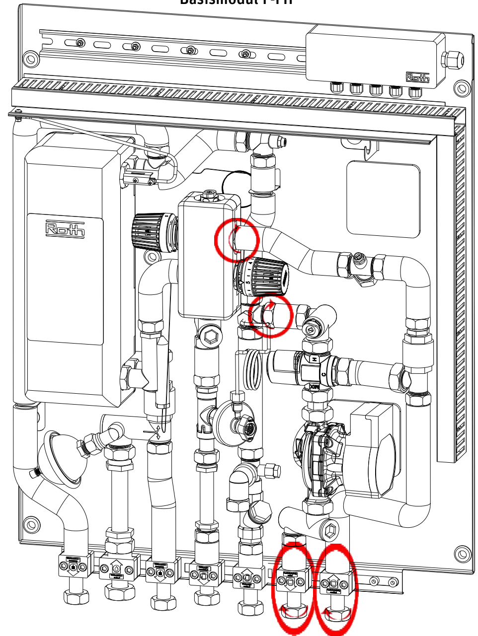
Basismodul F-FH
