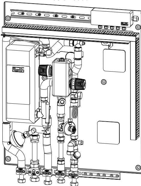
Basismodul F
