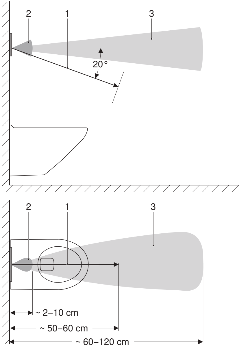
Şekil 1: Algılama alanları
