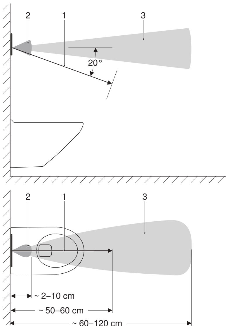
Slika 1: Območja zaznavanja
