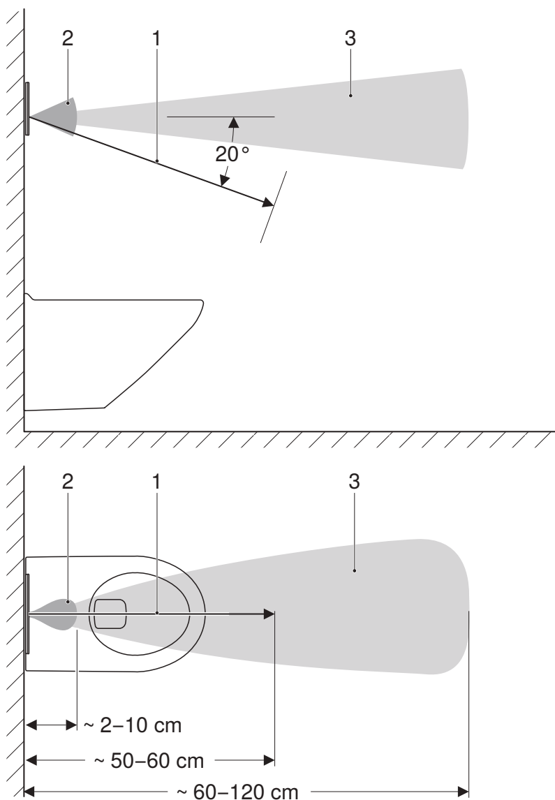
Afbeelding 1: Detectiebereiken
