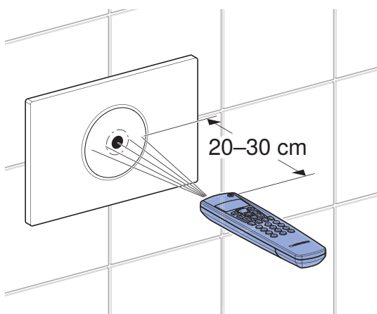
插图 2： 用 Geberit 服务遥控器进行操作
