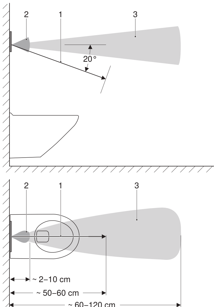
Obrázek 1: Snímací rozsahy
