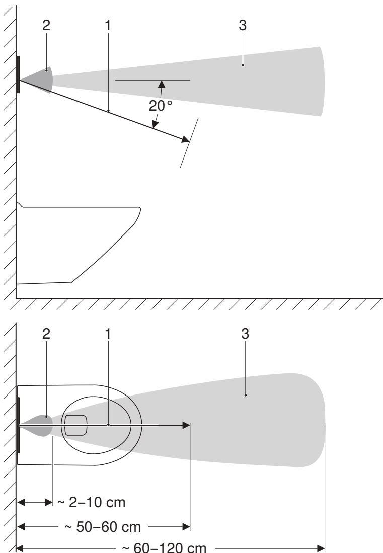
Figura 1: Campi rilevazione
