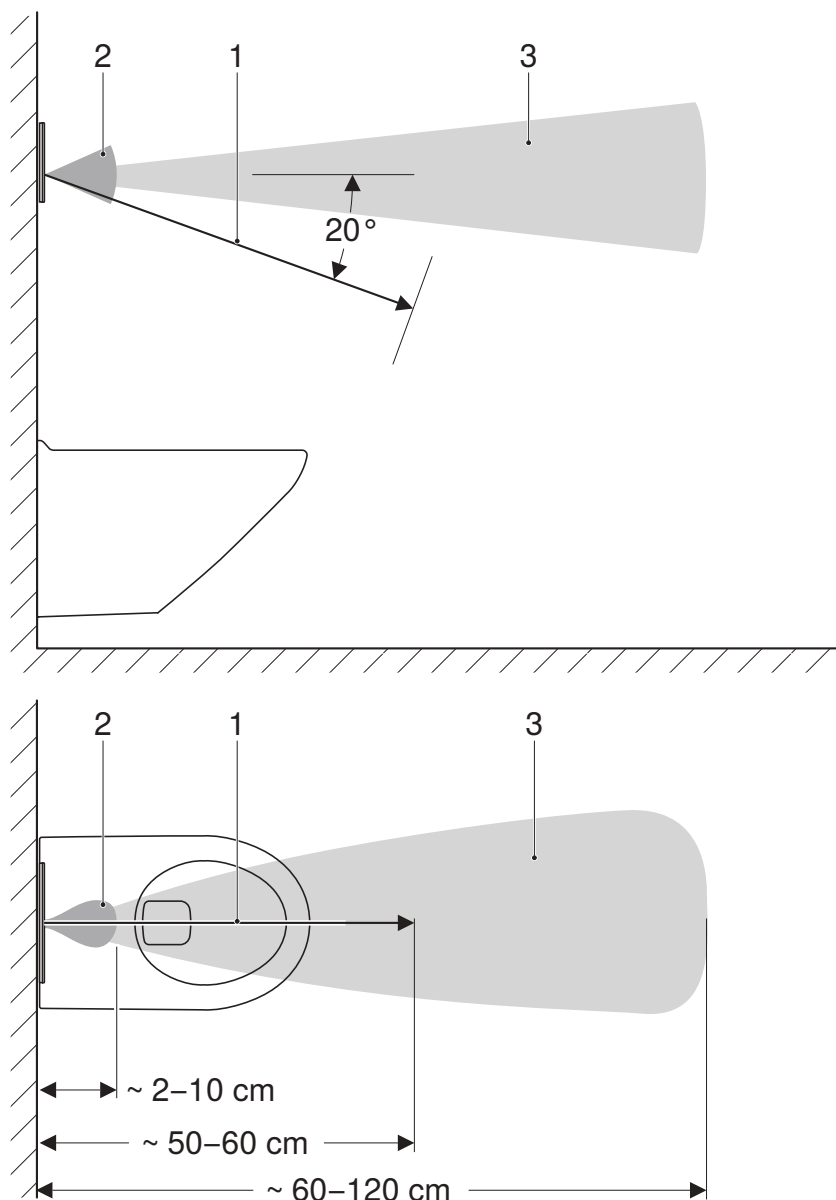
Kuva 1: Ilmaisualueet
