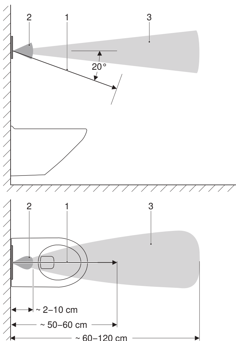
Εικόνα 1: Γωνίες ανίχνευσης
