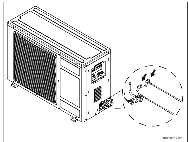
Bild 15 Verschraubung
