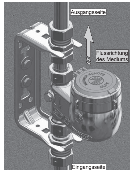
Montageschritt 7
