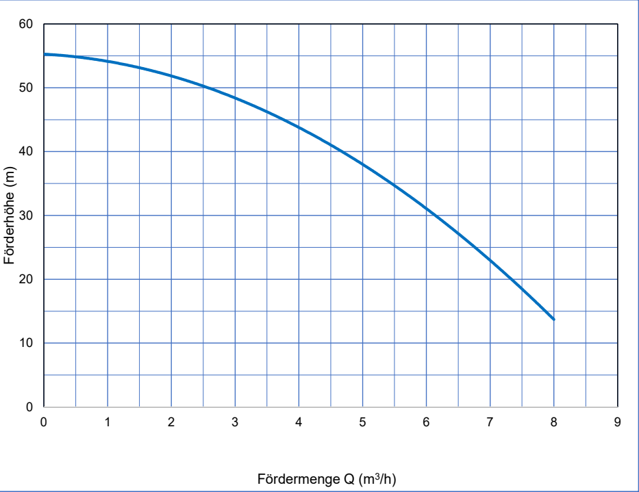
Technische Förderdaten
