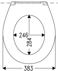
Gesamtlänge: 431 mm
