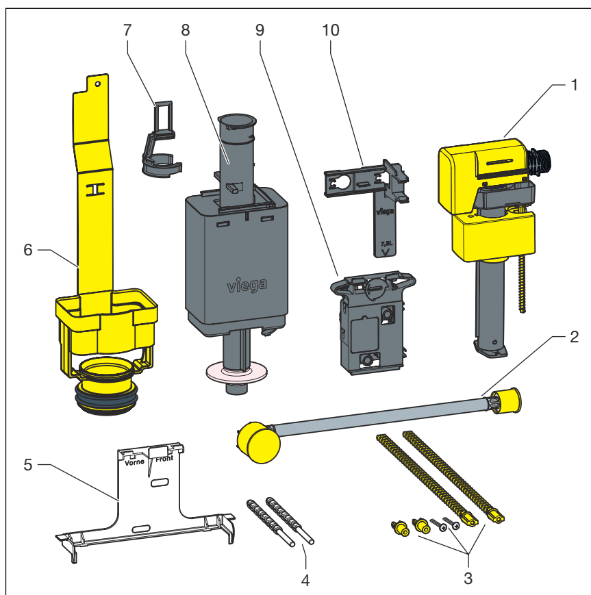
Abb. 1: Ersatzteilset
