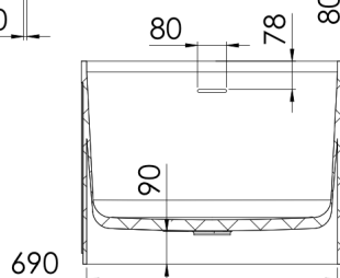
Schnitt B-B
