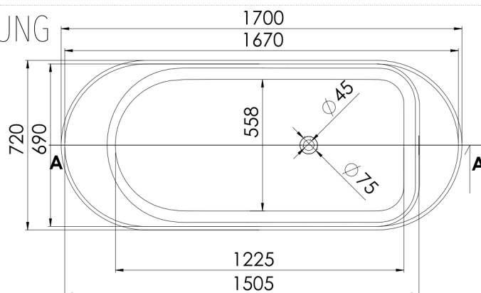
Schnitt A-A
