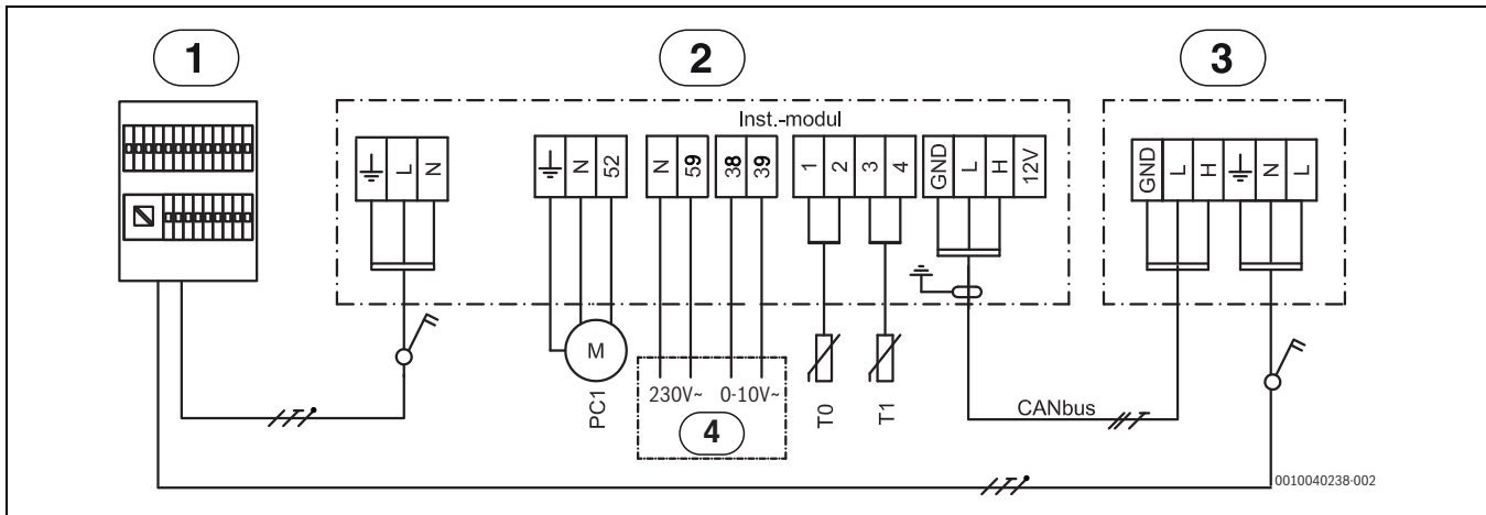
Bild 42 Schaltplan
