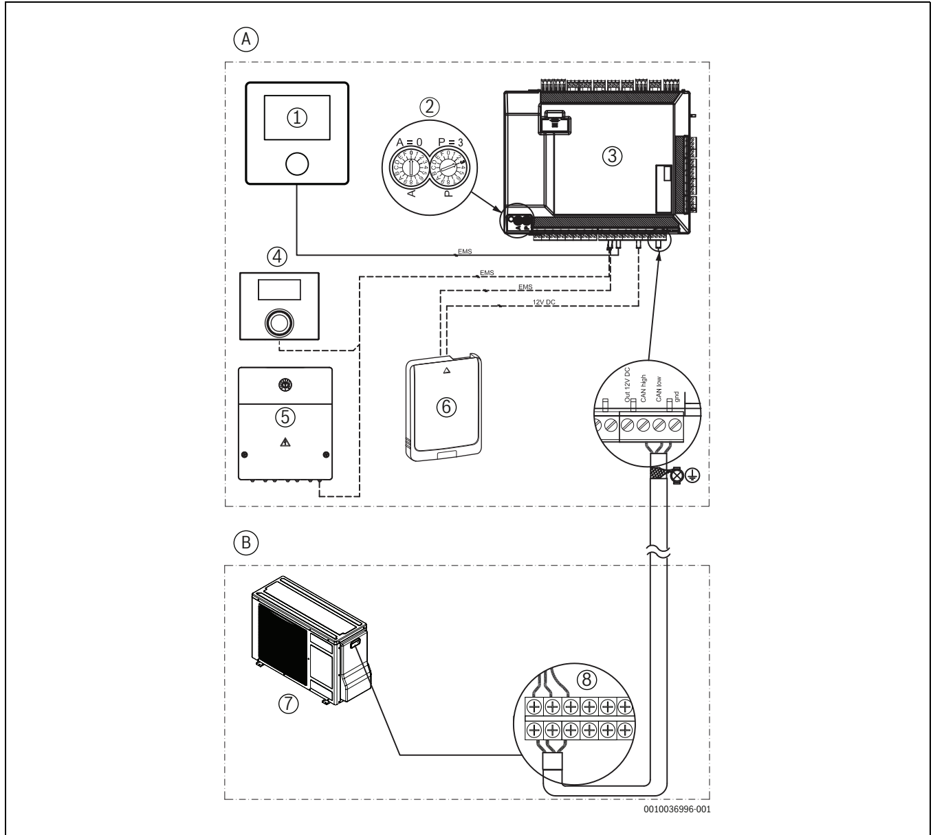
Bild 41 CAN und EMS Anschlüsse
