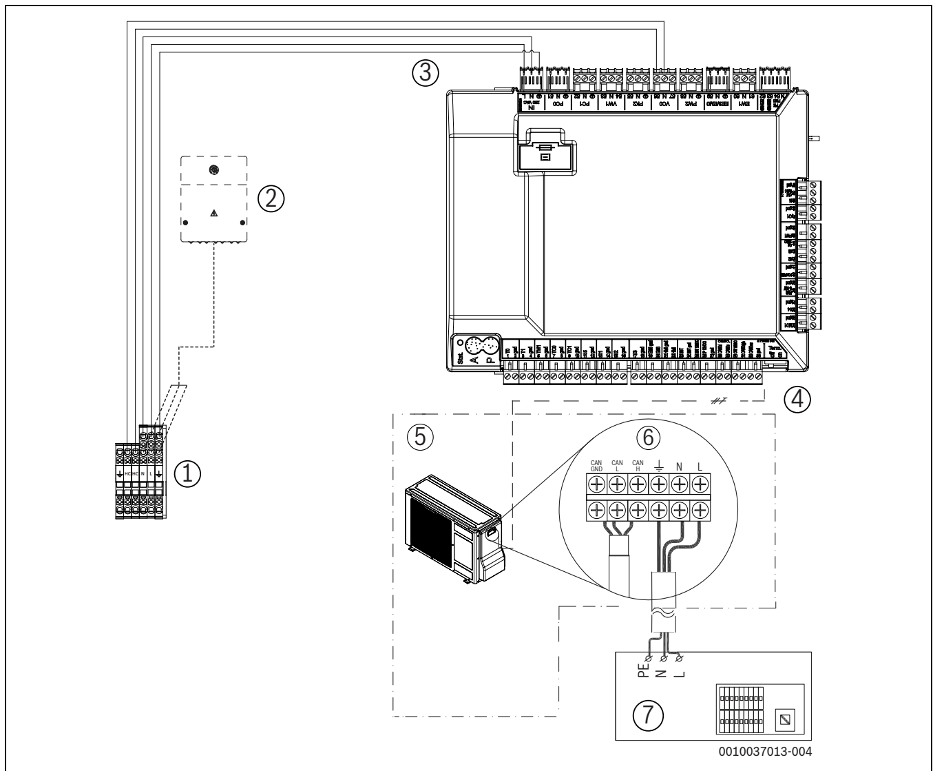
Bild 43 Inneneinheit mit 230 V~ Außeneinheit
