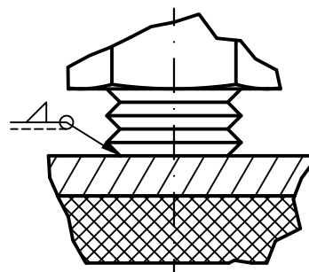
DETAIL Z Maßstab: 2:1
