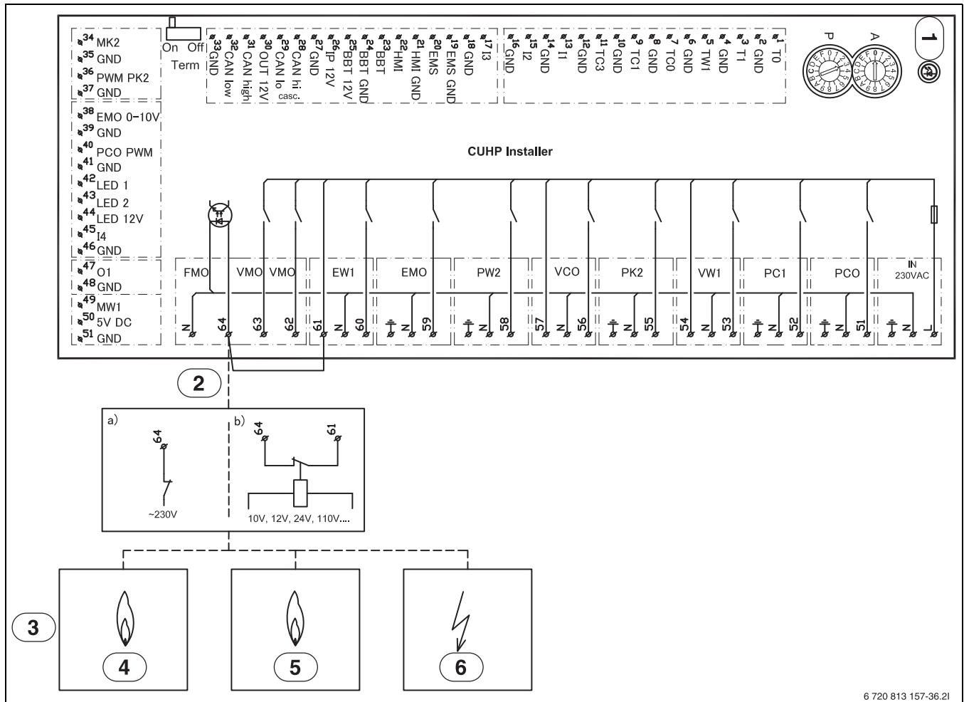
Bild 14 Schaltschema des Installationsmoduls, Alarm für externen Zuheizier
