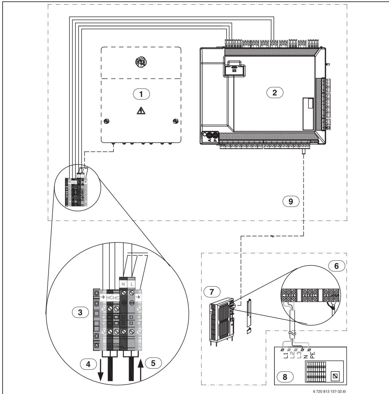
Bild 34 Inneneinheit mit 230V~ 1N Außeneinheit
