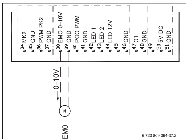
Bild 16 0- bis 10-V-Ansteuerung für externe Zuheizers
