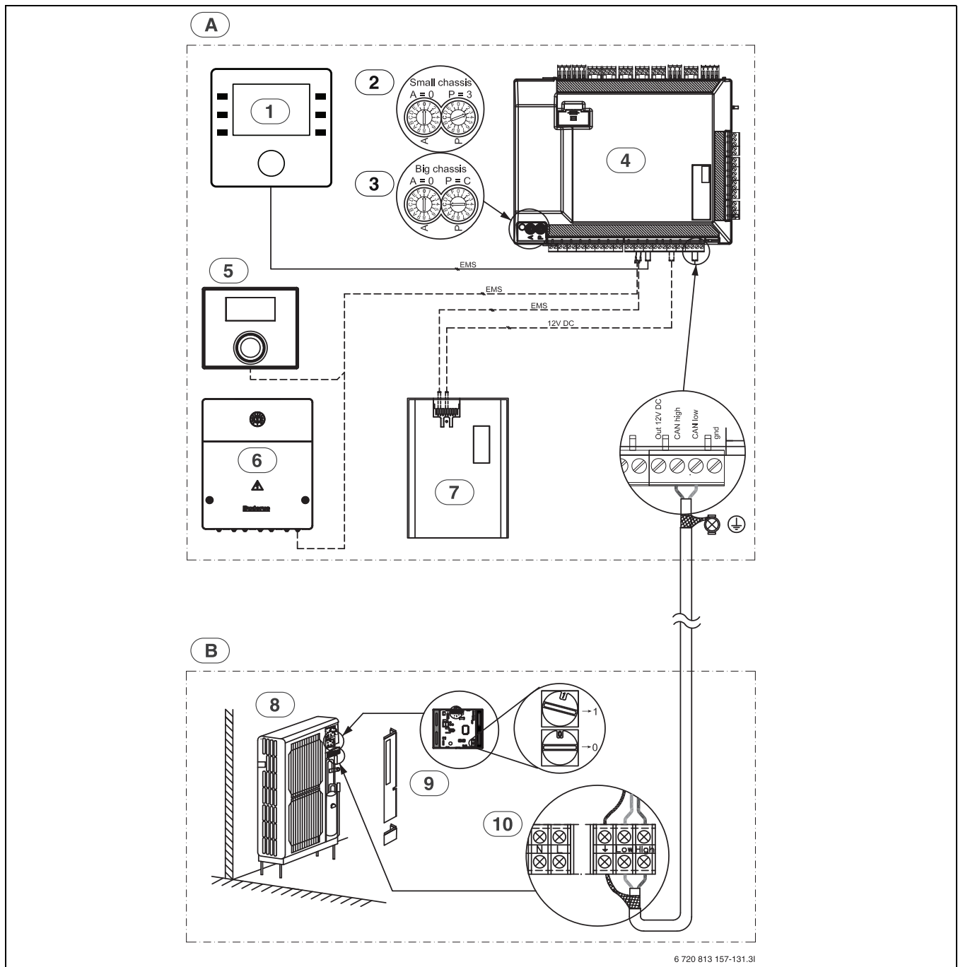
Bild 33 Übersicht der Inneneinheit mit externem Zuheizer
