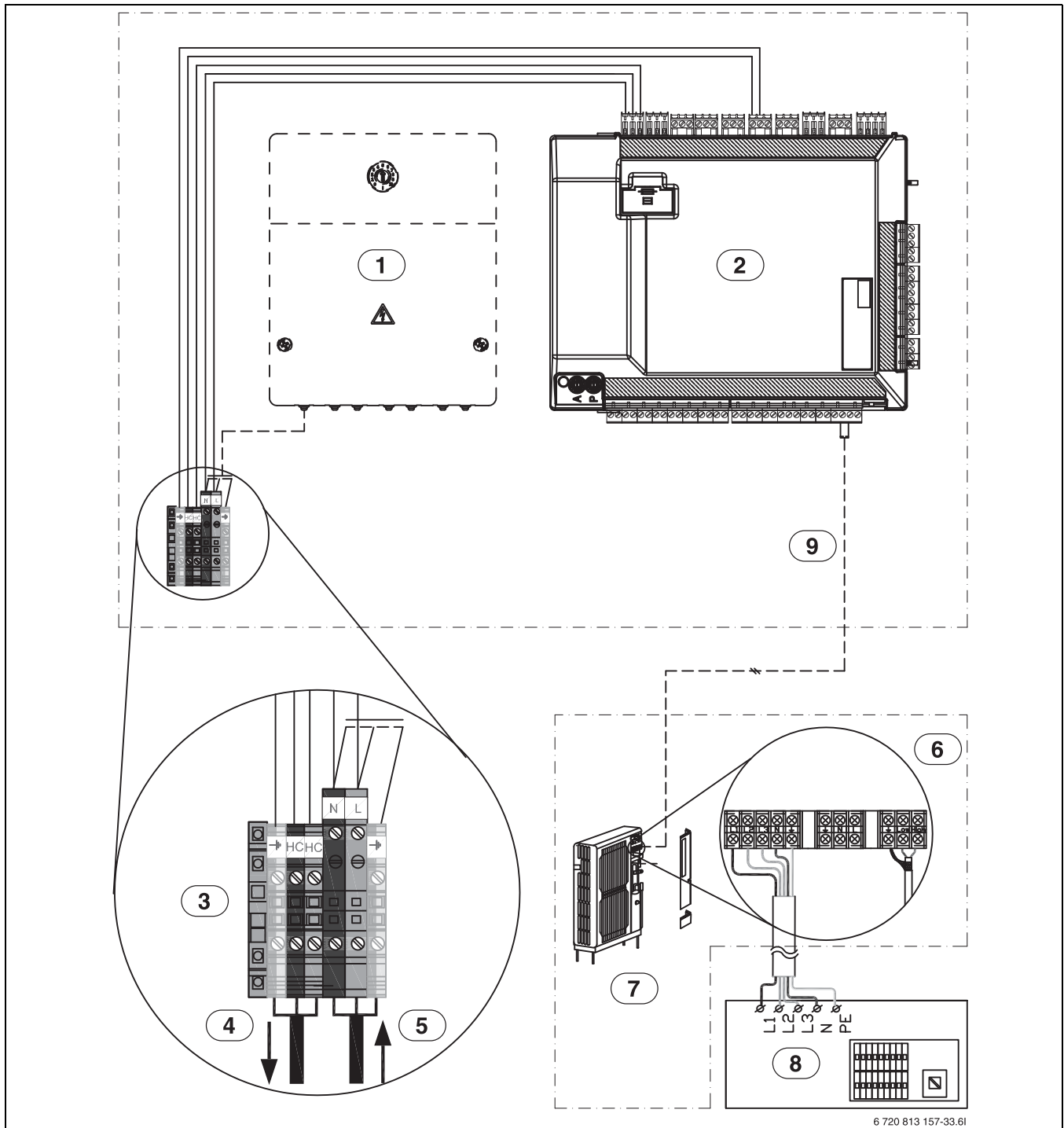
Bild 35 Inneneinheit mit 400V~ 3N Außeneinheit
