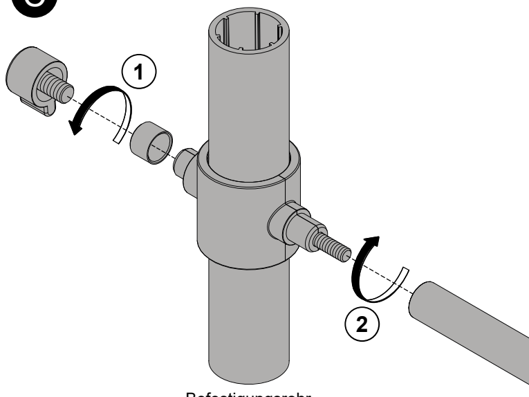
Befestigungsrohr Tube OUTside
