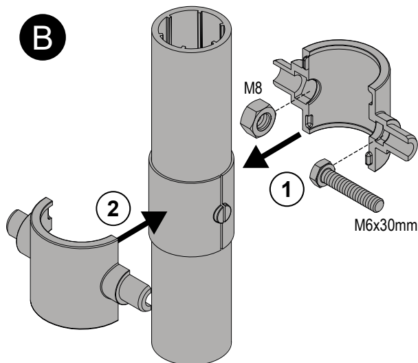
Befestigungsrohr Tube OUTside
